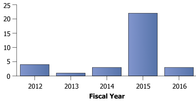
Forcible Rape
